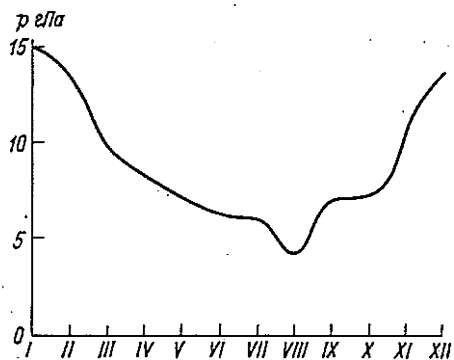
Рис. 8. Амплитуда колебаний среднего месячного атмосферного давления p .
