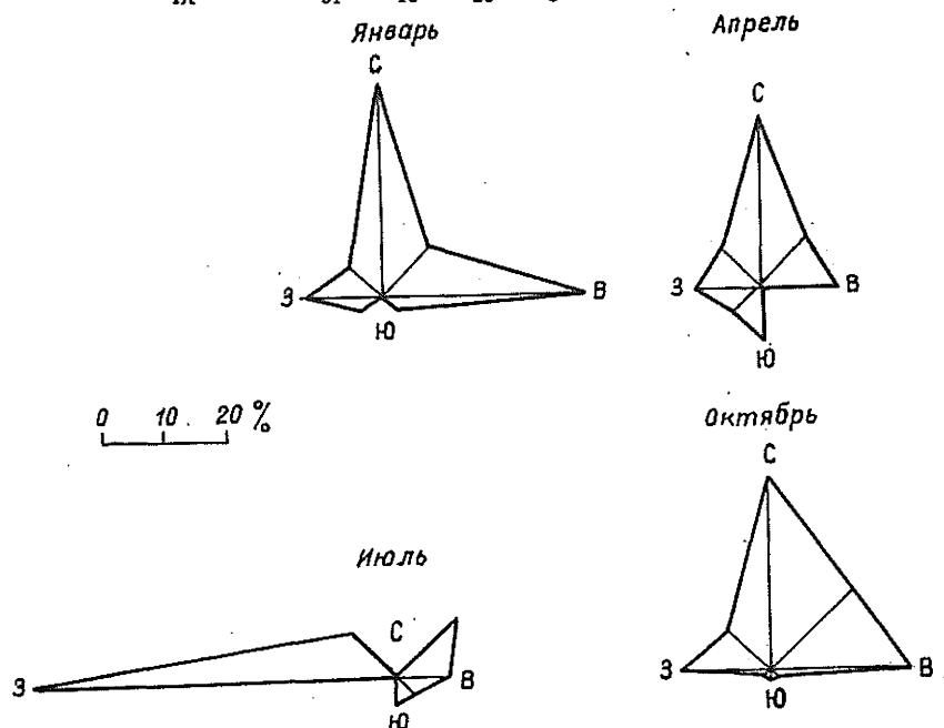
Рис. 34. Повторяемость (%) дальности видимости 4 км и менее при различных направлениях ветра.
