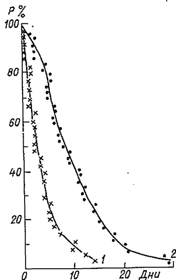
Рис. 35. Интегральные кривые среднего за год числа дней с гололедом (1), изморозью (2) различной вероятности ( P ) выше указанных пределов.
