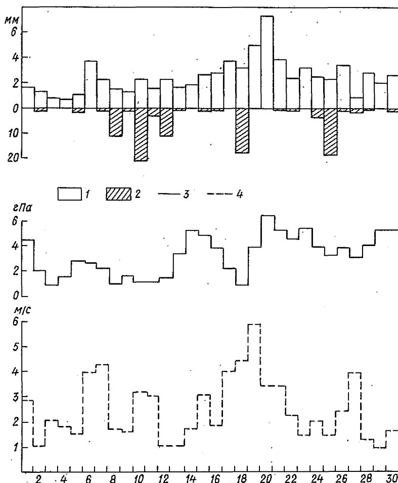
Рис. 1. Хронологический график за апрель 1980 г. Ст. Озерная. Водоиспарительная площадка II типа.
