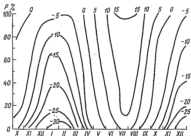
Рис. 17. Изоплеты абсолютного минимума температуры воздуха (°C) различной вероятности P.
