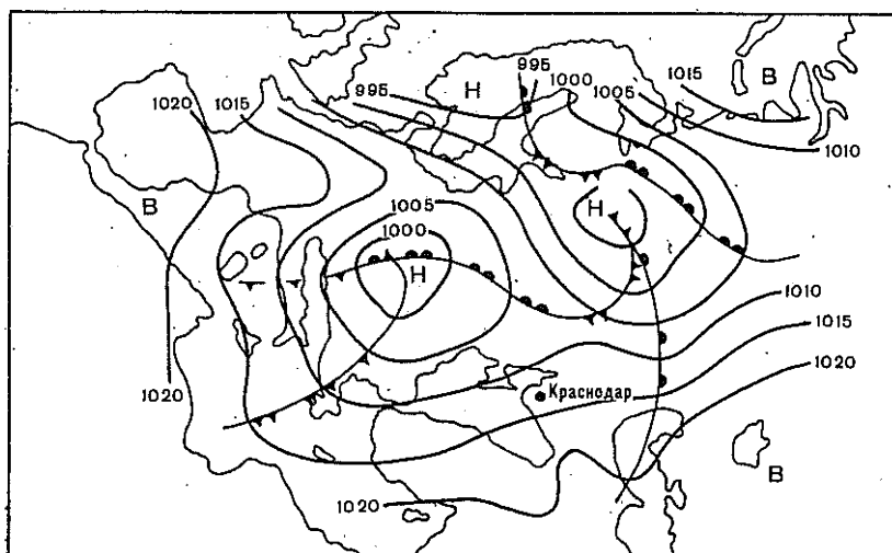
Рис. 7. Карта погоды за 3 ч 24 февраля 1966 г. (условия интенсивного потепления).
