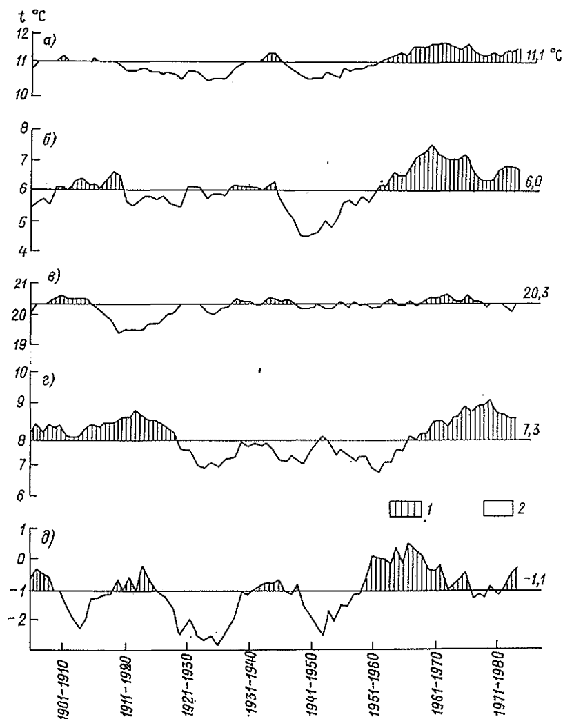
Рис. 38. Средняя температура воздуха по сезонам и за год (скользящие десятилетия).
