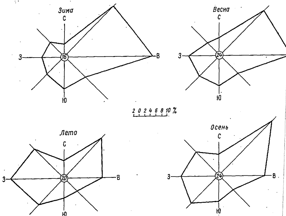
Рис. 12. Повторяемость (%) направлений ветра в различные сезоны года и число дней со штилем (цифра в кружке). Краснодар, Белозерный.
