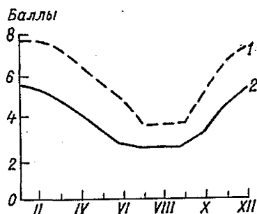
Рис. 28. Годовой ход облачности (баллы). 1 – общая облачность, 2 – нижняя облачность.
