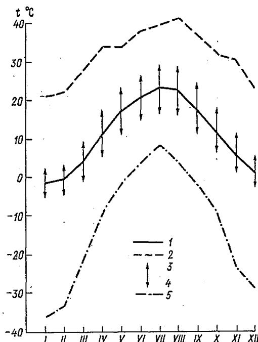
Рис. 13. Годовой ход температуры воздуха t .
