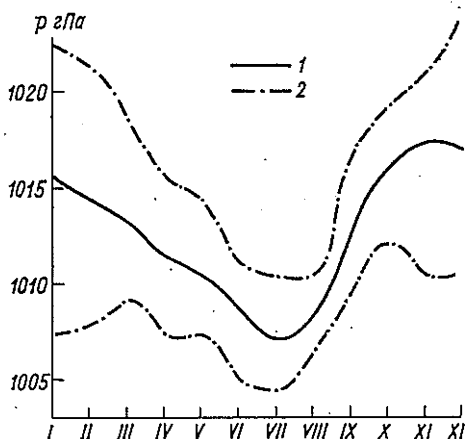
Рис. 9. Годовой ход среднего месячного атмосферного давления p (на уровне барометра станции).
