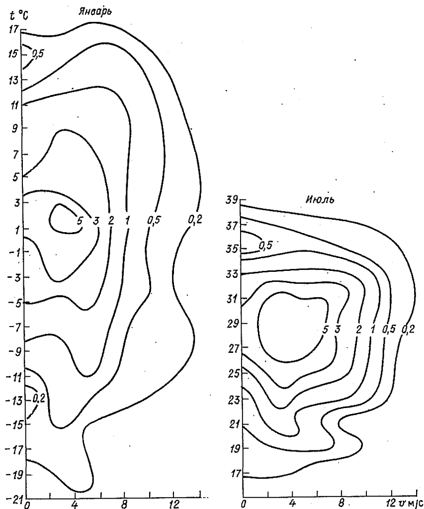
Рис. 19. Повторяемость (%) различных сочетаний температуры воздуха t и скорости ветра v в 13 ч.
