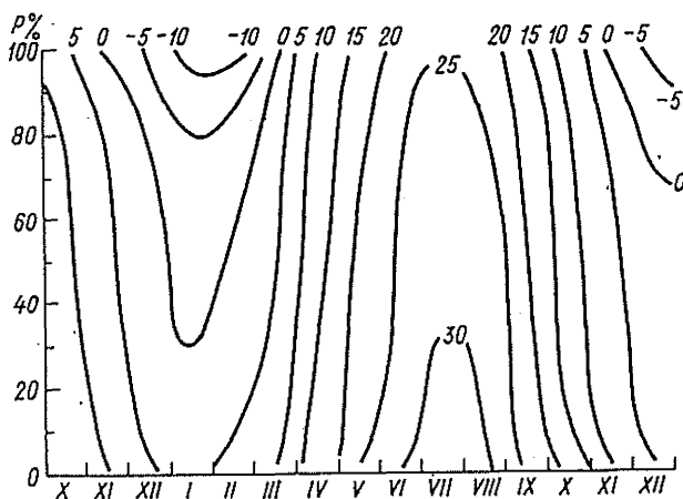
Рис. 22. Изоплеты средней месячной температуры поверхности почвы ( ^{\circ}\text{C} ) различной вероятности P .
