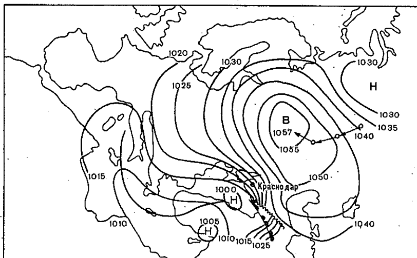
Рис. 6. Карта погоды за 15 ч 5 января 1969 г. (условия возникновения сильной пыльной бури).
