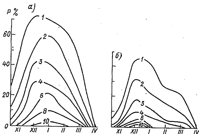
Рис. 36. Изоплеты числа дней с изморозью (а) и гололедом (б) различной вероятности ( P ) выше указанных пределов.
