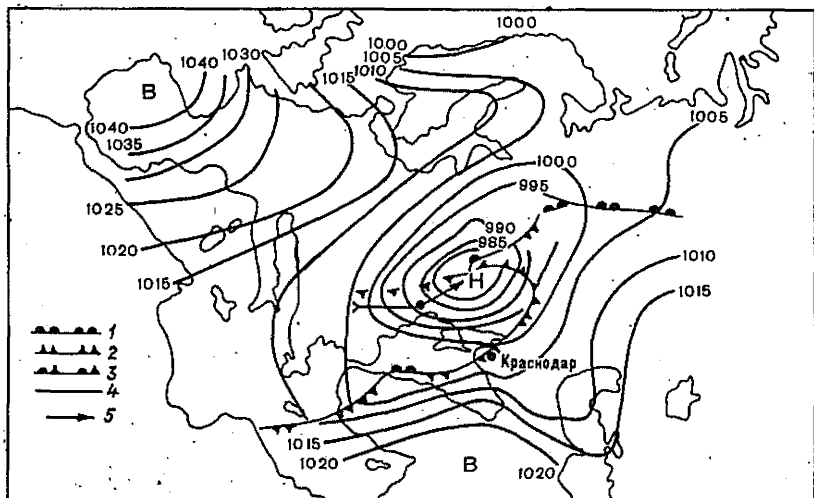
Рис. 4. Карта погоды за 15 ч февраля 1962 г. (условия возникновения сильного ветра и фёна).
