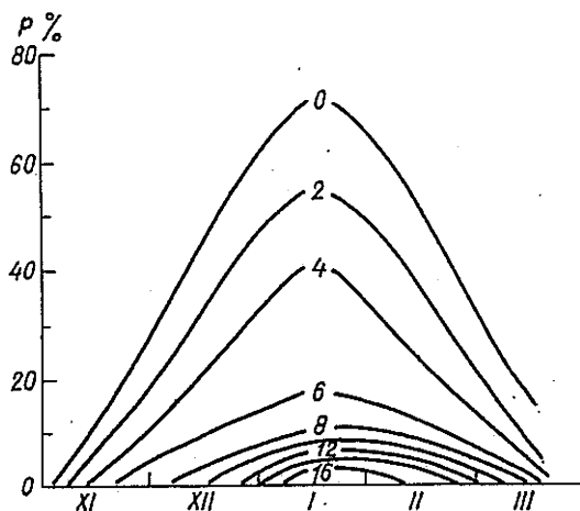
Рис. 15. Изоплеты числа дней со средней суточной температурой воздуха -10^{\circ}\text{C} и ниже различной вероятности P .
