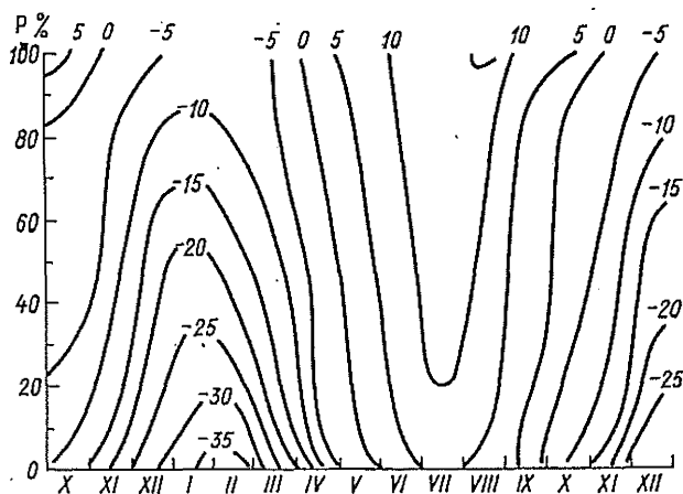
Рис. 23. Изоплеты абсолютного минимума температуры поверхности почвы ( ^{\circ}\text{C} ) различной вероятности P .
