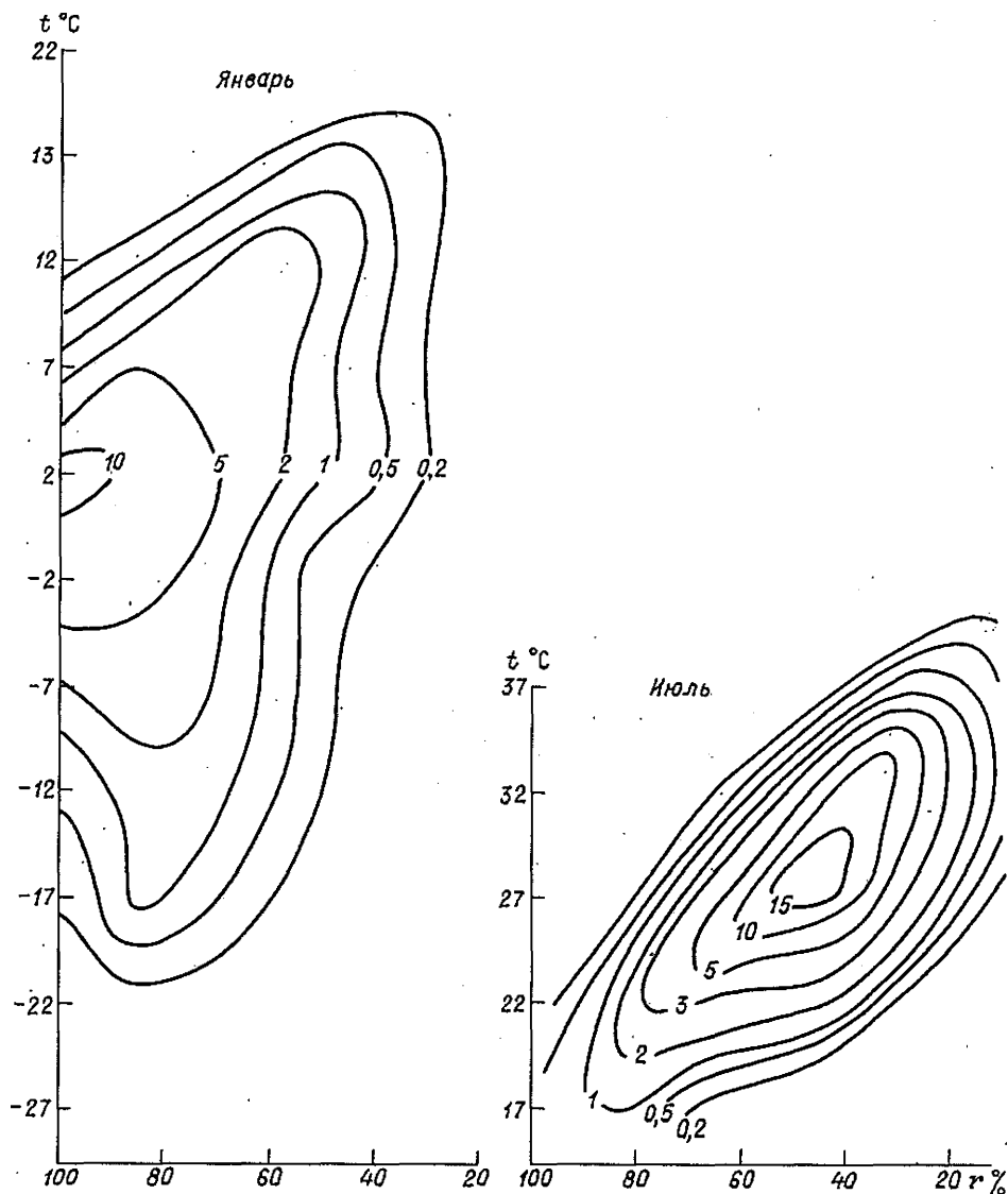
Рис. 20. Повторяемость (%) различных сочетаний температуры воздуха t и относительной влажности r .
