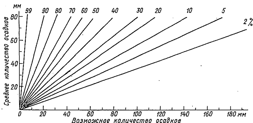
Рис. 26. Номограмма для расчета количества осадков различной обеспеченности (%).
