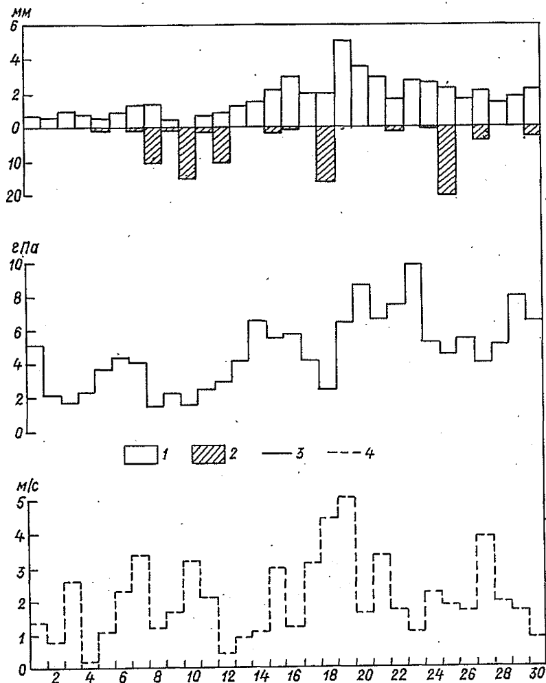
Рис. 2. Хронологический график за апрель 1980 г. Ст. Краснодар, Круглик. Водоспарительная площадка III типа.
