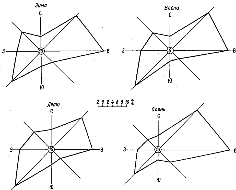
Рис. 11. Повторяемость (%) направлений ветра в различные сезоны года и число дней со штилем (цифра в кружке). Краснодар, Пашковская.
