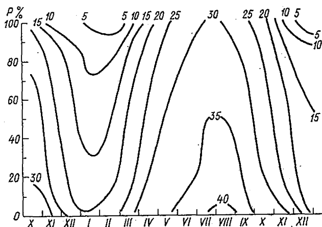
Рис. 18. Изоплеты абсолютного максимума температуры воздуха (°С) различной вероятности P .
