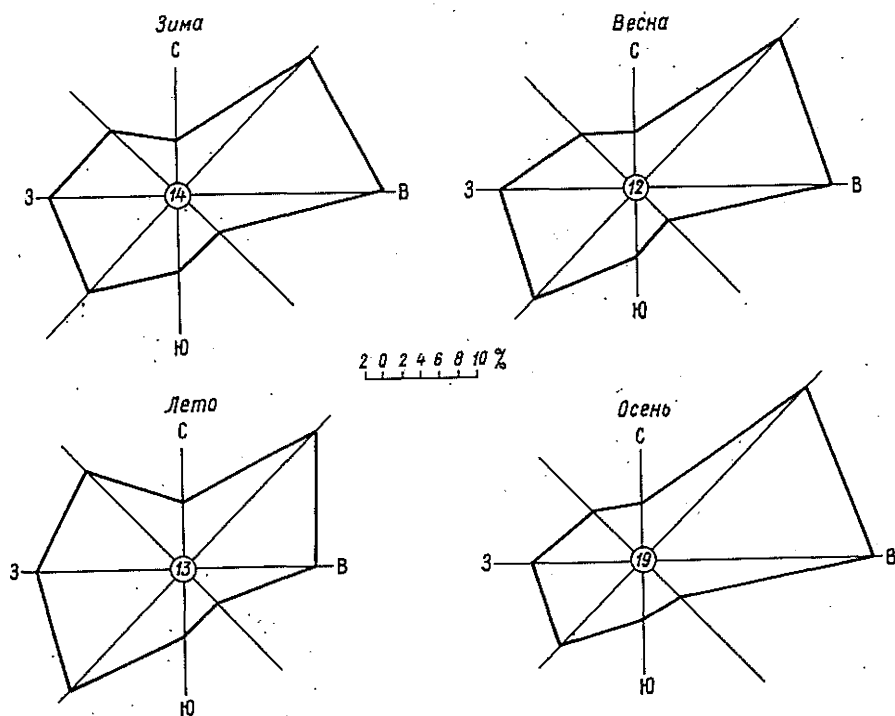
Рис. 10. Повторяемость (%) направлений ветра в различные сезоны года и число дней со штилем (цифра в кружке). Краснодар, Круглик.
