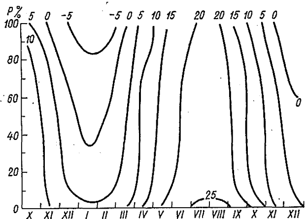
Рис. 14. Изоплеты средней месячной температуры воздуха (°C) различной вероятности P .
