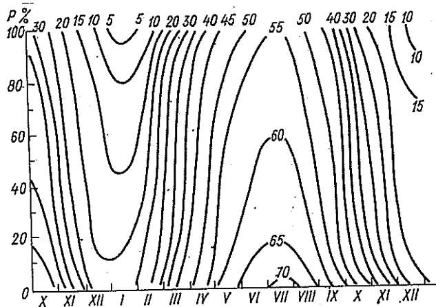
Рис. 24. Изоплеты абсолютного максимума температуры поверхности почвы (°С) различной вероятности P .
