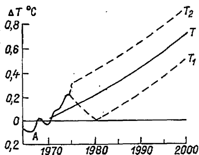
Рис. 40. Прогноз изменений температуры воздуха.
