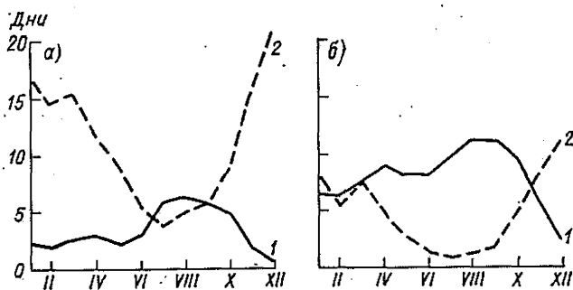
Рис. 30. Годовой ход числа ясных (1) и пасмурных (2) дней по общей (а) и нижней (б) облачности.
