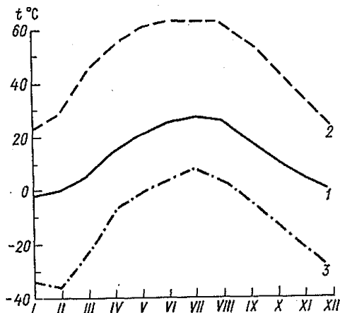
Рис. 21. Годовой ход температуры поверхности почвы. 1 – средняя месячная, 2 – абсолютный максимум, 3 – абсолютный минимум.
