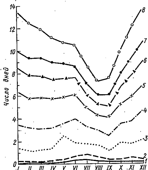
Рис. 27. Число дней с различным количеством осадков.
