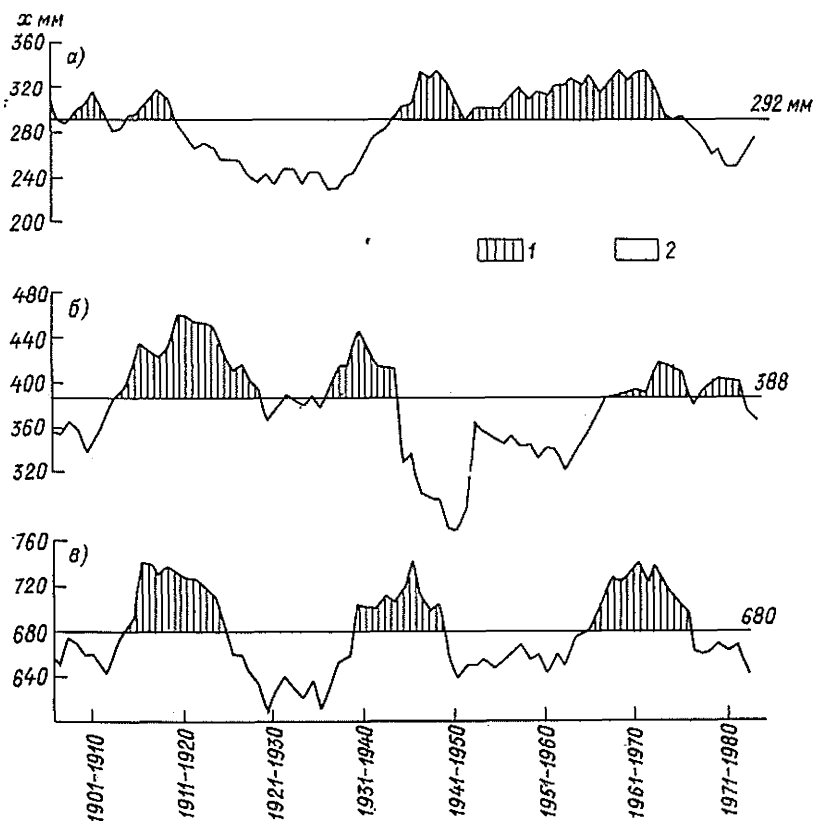
Рис. 39. Среднее количество осадков (скользящие десятилетия).
