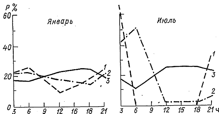
Рис. 32. Повторяемость ( P ) дальности видимости в различные часы суток. 1) 1 км и менее; 2) 4 км и менее; 3) 4 км и более.
