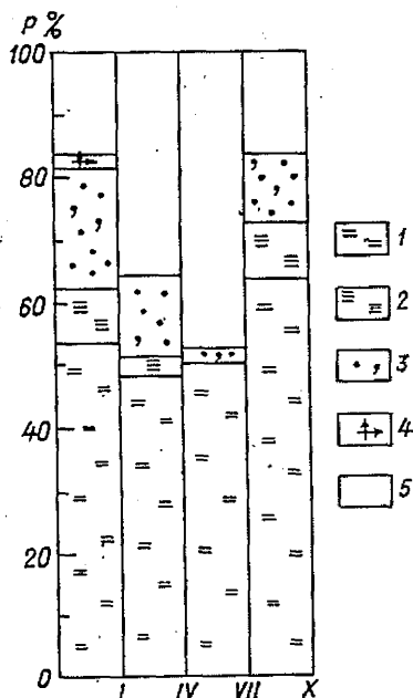
Рис. 33. Повторяемость ( P ) по сезонам атмосферных явлений при дальности видимости 4 км и менее.
