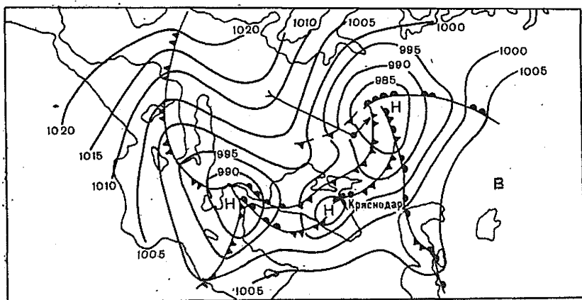
Рис. 5. Карта погоды за 9 и 12 марта 1968 г. (условия формирования сильных осадков).
