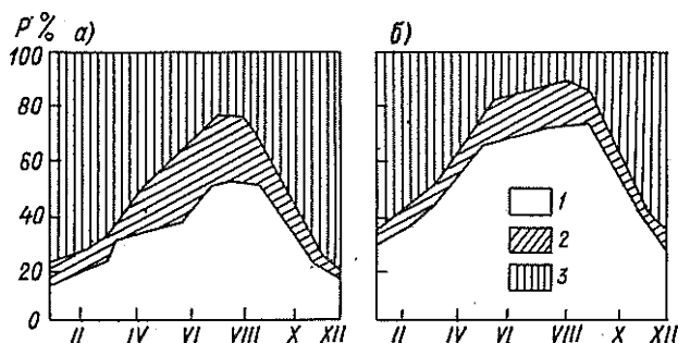
Рис. 29. Вероятность P ясного (1), полужасного (2) и пасмурного (3) состояния неба по общей (а) и нижней (б) облачности.
