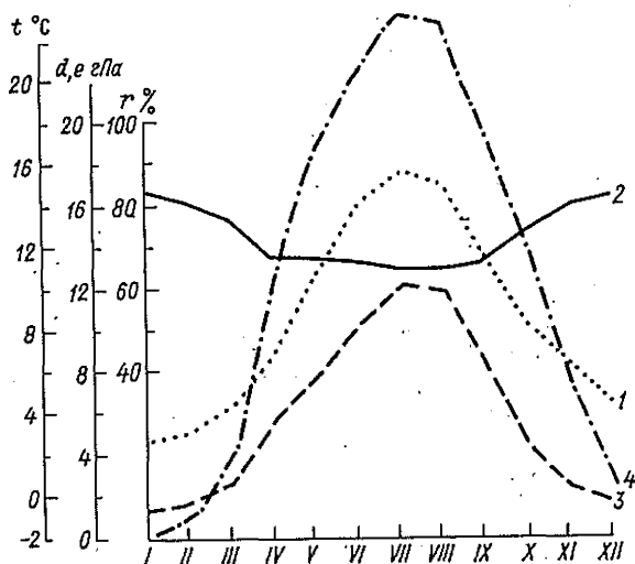
Рис. 25. Годовой ход характеристик влажности и температуры воздуха.
