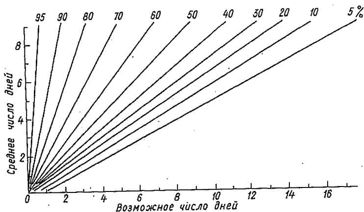
Рис. 31. Номограмма для расчета среднего месячного числа дней с туманом различной обеспеченности (%).
